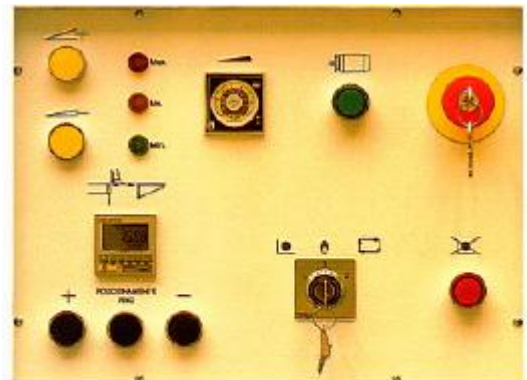
Cuadro de mandos standard con botones pulsadores para regulación del ángulo de corte y del tope trasero, con selector del ciclo de funcionamiento y con temporizador de la longitud de corte.
